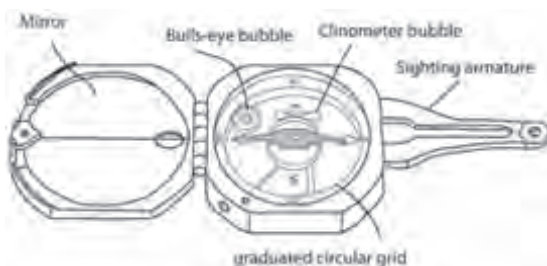
Fig. 4.7: Brunton Compass
