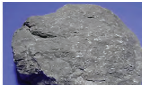
Fig.1.14: Basalt
