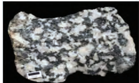
Fig.1.11: Diorite
