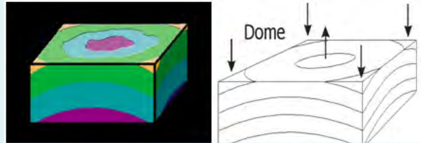
Fig. 4.20: Dome
