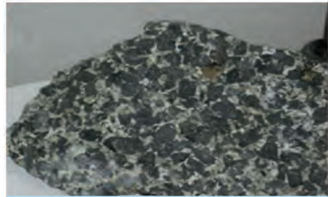
Fig.1.13: Gabbro
